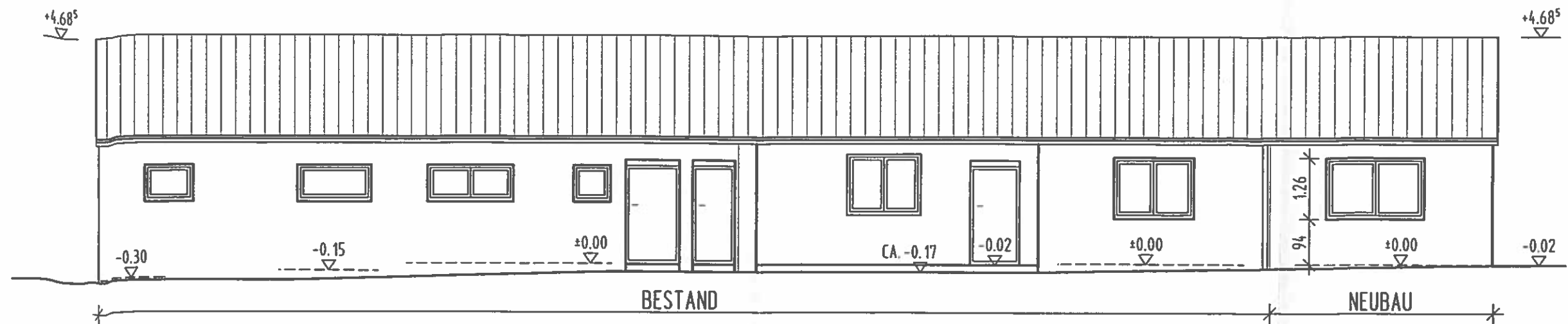
VORDERANSICHT
