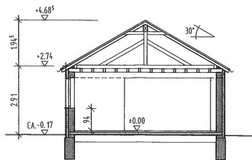
SCHNITT B-B
