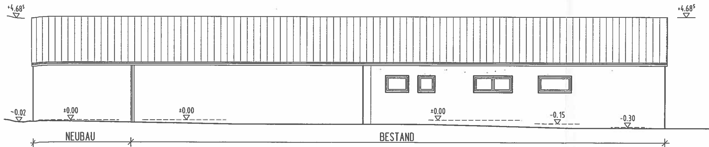
RÜCKANSICHT
