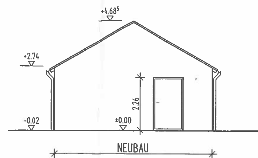
SEITENANSICHT
