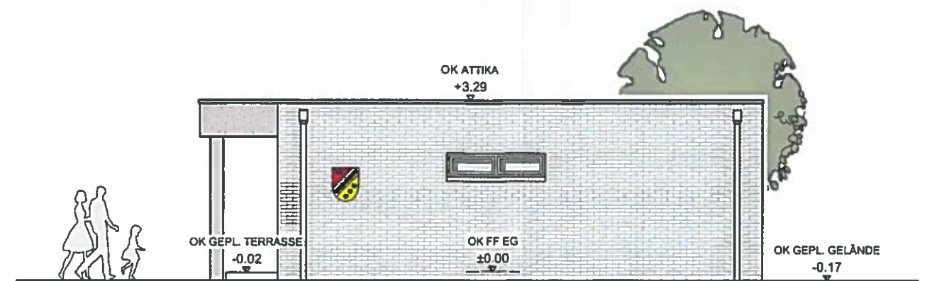
RECHTE SEITENANSICHT
