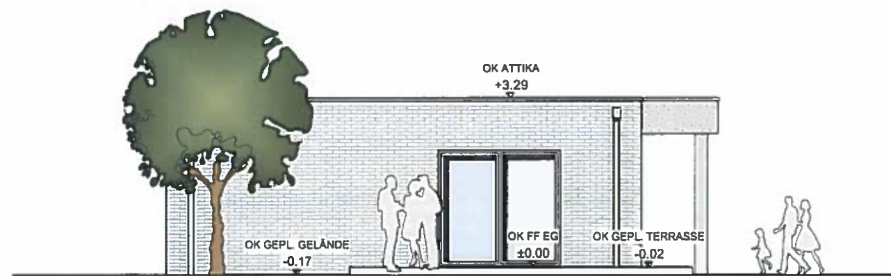
LINKE SEITENANSICHT
