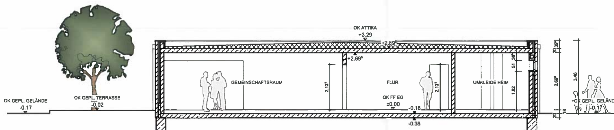
SCHNITT A-A
