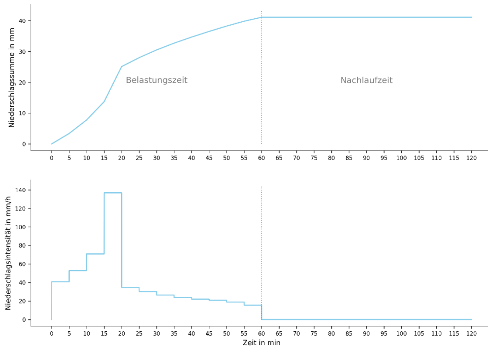
Abbildung 4-5: Euler Typ II Verteilung des Niederschlags N30
