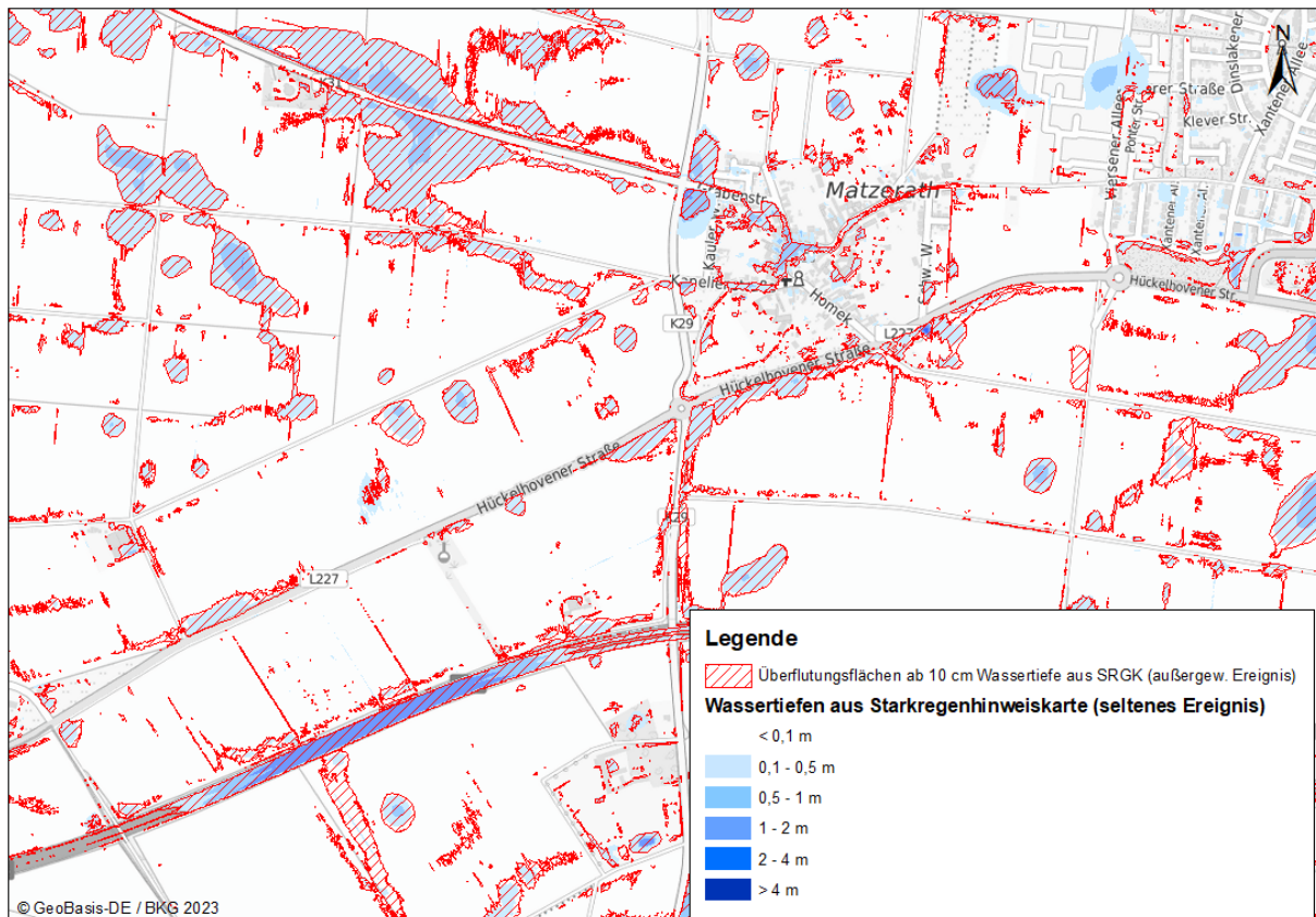
Abbildung 4-9: Beispiel für Abgleich Überflutungsflächen für das außergewöhnliche Ereignis aus den SRGK mit denen der BKG-Starkregenhinweiskarten
