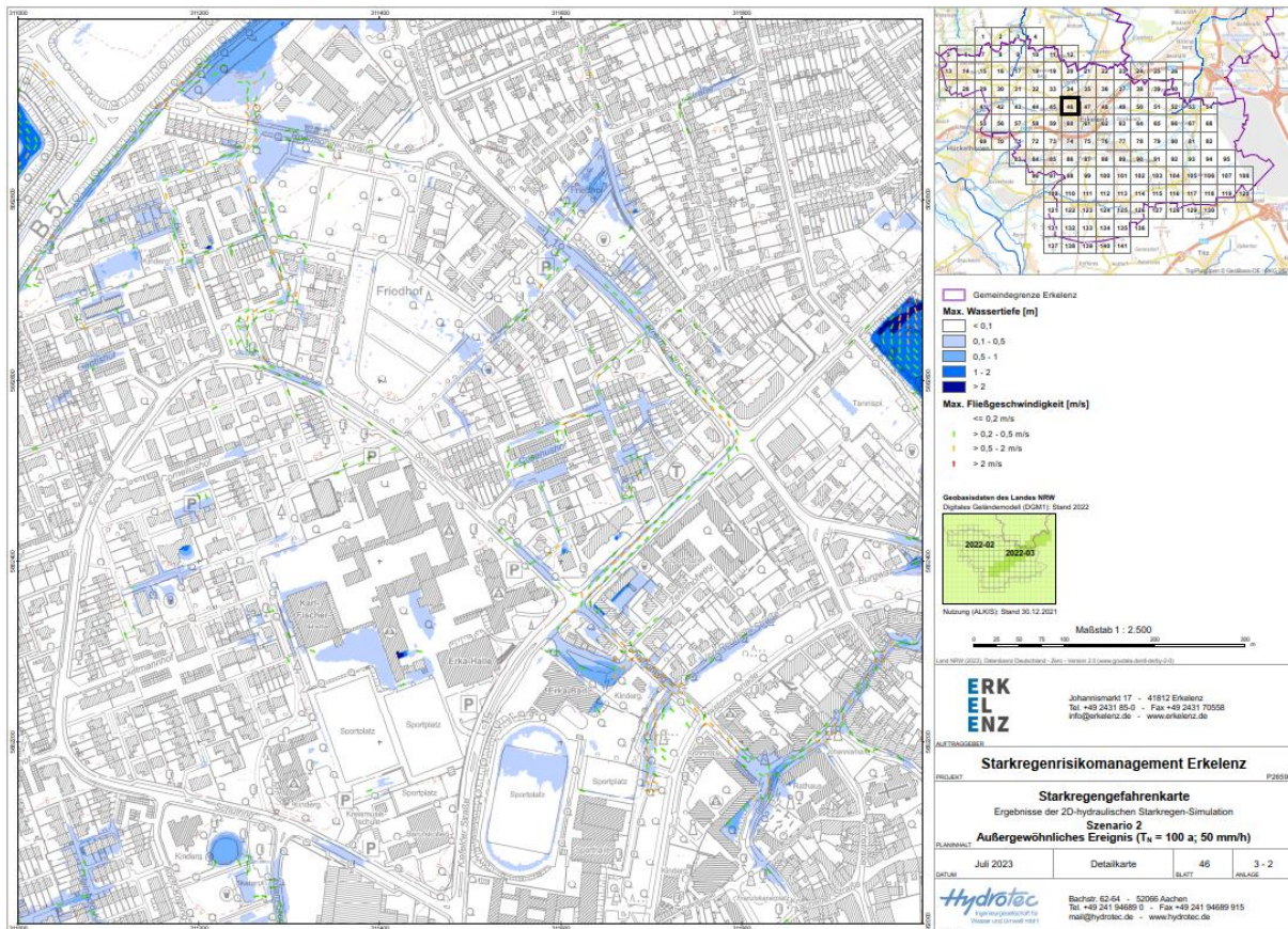
Abbildung 4-7: Detaildarstellung der maximalen Überflutungsausdehnung und der maximalen Überflutungstiefe je Niederschlagsszenario, hier für das außergewöhnliche Szenario ( T_n = 100 a; 50 mm/h)
