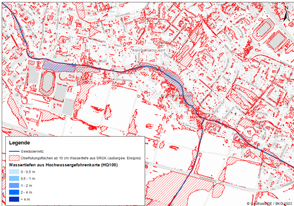
Abbildung 4-10: Darstellung Überflutungsflächen der HWGK (HQ100) und der SRGK (außergewöhnliches Ereignis)
