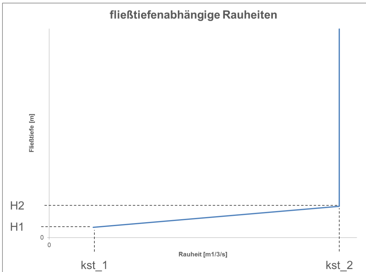
Abbildung 4-3: Ansatz zur Ermittlung von fließtiefenabhängigen Rauheiten mit H1 = 2 \text{ cm} , H2 = 10 \text{ cm} , kst\_1 und kst\_2 entsprechend Tabelle 4-1
