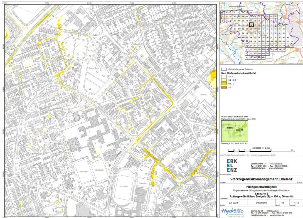
Abbildung 4-8: Detaildarstellung der maximalen Fließgeschwindigkeiten je Niederschlags-szenario, hier für das außergewöhnliche Szenario ( T_n = 100 a; 50 mm/h)
