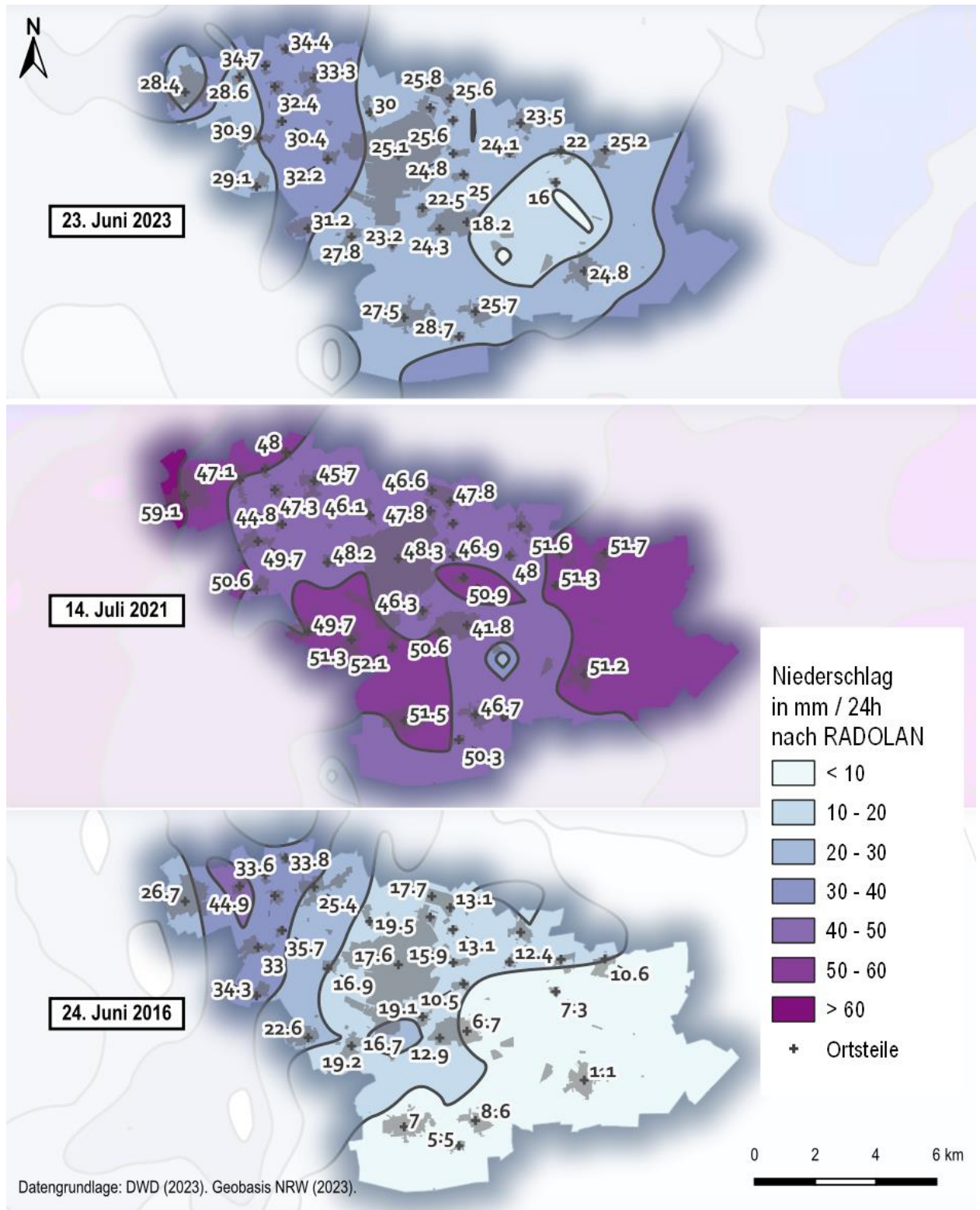
Abbildung 25: Modellierte Niederschlagsmengen für drei ausgewählte Ereignisse auf dem Erkelenser Stadtgebiet.
